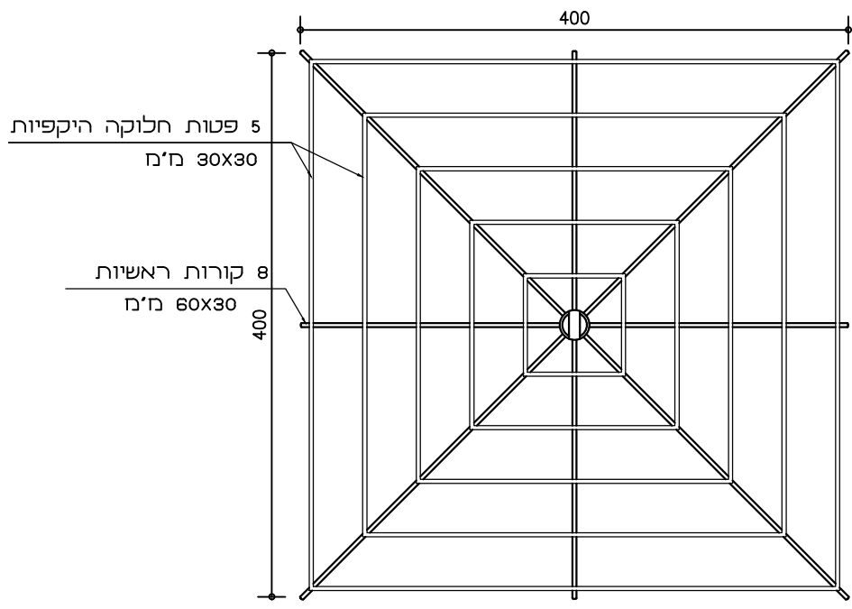
תכנית קירוי סככה- פלדה ק.מ. 1:50
