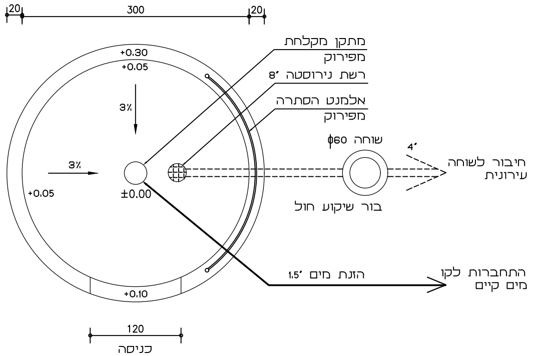
תכנית מקלחת חוף קנ"מ 1:50
